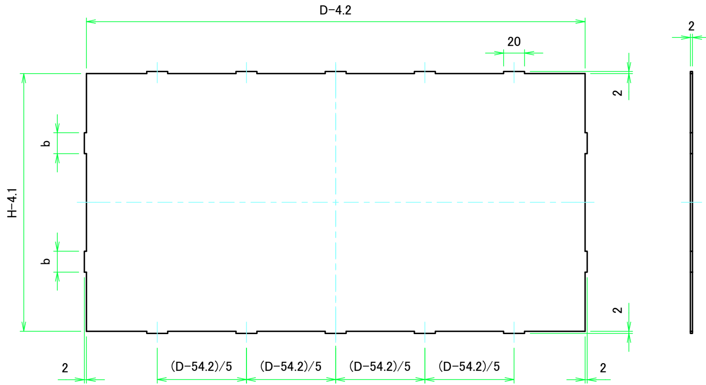
Dパネル1表面 / D panel 1 Frontside
